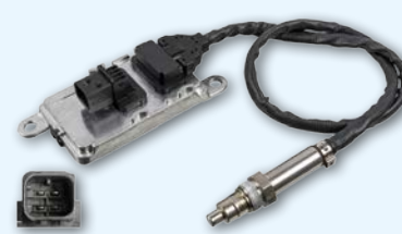
⌘ ArtikelNr. 176854 NOX- SENSOR – Vor-Kat – Mercedes Benz 010 153 14 28
